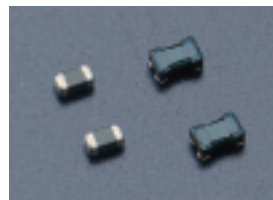
(左)チップフェライトビーズ (右)チップ共通モードチョークコイル
